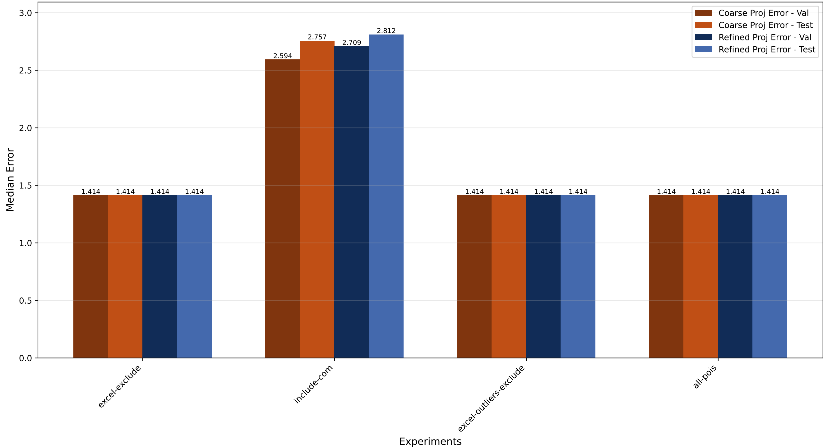
Error Type Comparison - MedianError (Coarse Proj vs Refined Proj)
