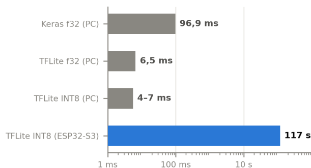
Figura 5. Tempo de inferência do mesmo modelo em cada plataforma (escala logarítmica). O arquivo INT8 é idêntico no PC e na ESP32-S3.
