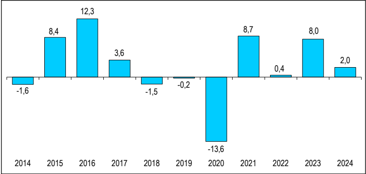
VALOR AGREGADO BRUTO DE EXTRACCIÓN DE PETRÓLEO, GAS, MINERALES Y SERVICIOS CONEXOS, 2014-2024 (Variación porcentual anual)
