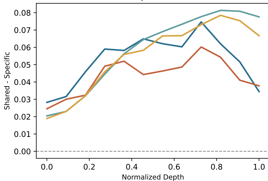
pSTG
