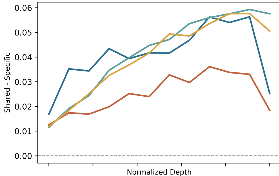
pSTG
