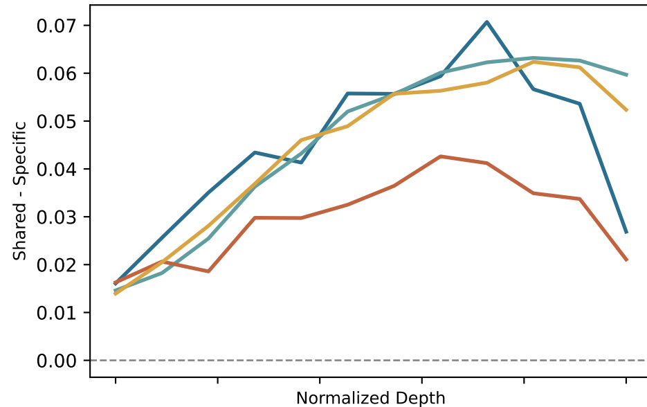
Heschl
