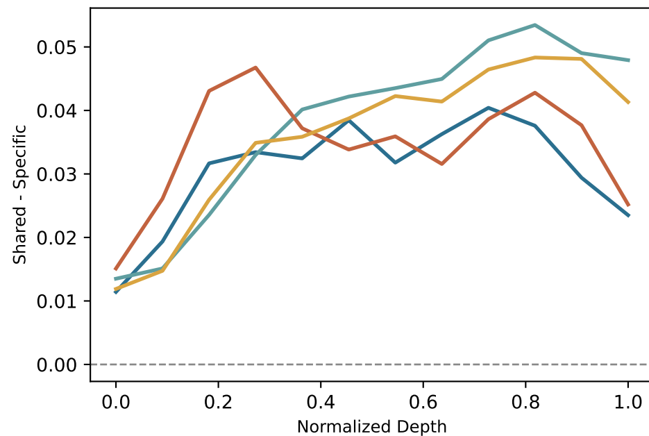
Heschl
