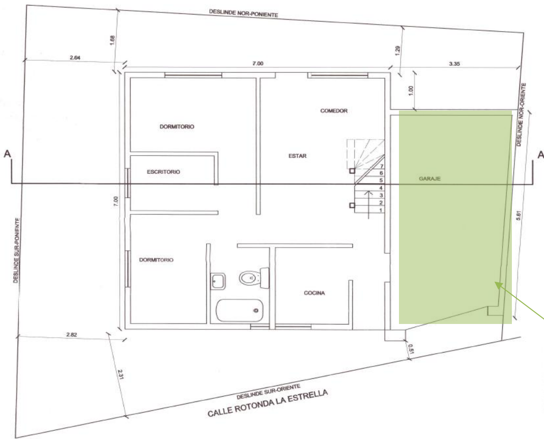
PLANTA DE ARQUITECTURA Y EMPLAZAMIENTO ESC.1/50
