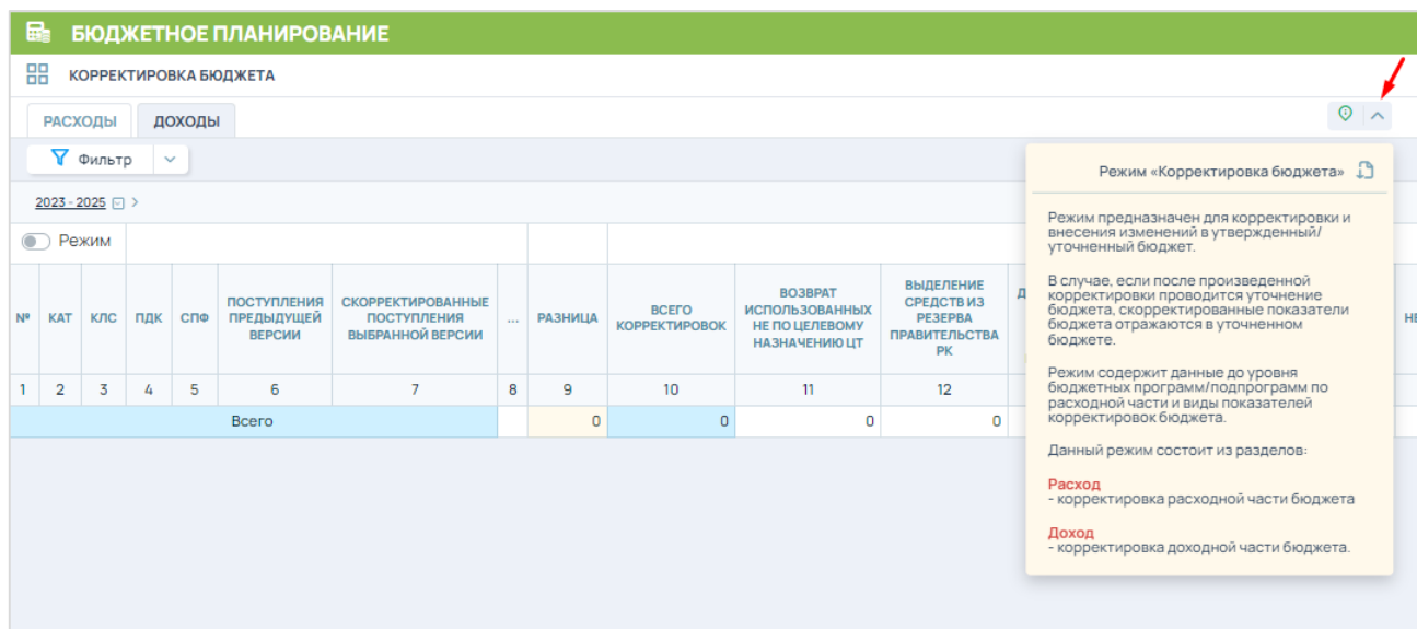
Рис.3.1.1 Функция «Информация»
