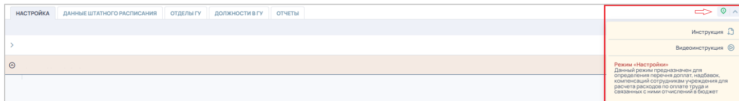
Рис. 3.1.2 Функция «Информация»
