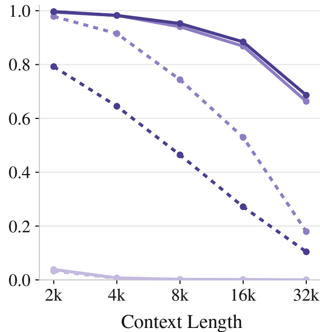
QDmatch (NQ)
