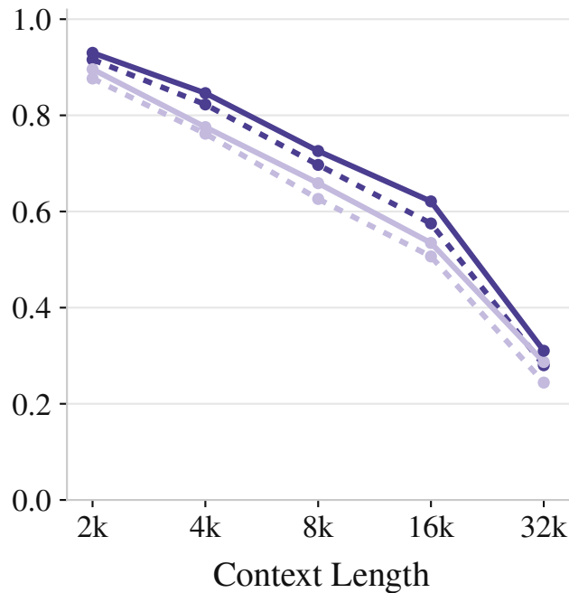
BEIR FiQA
