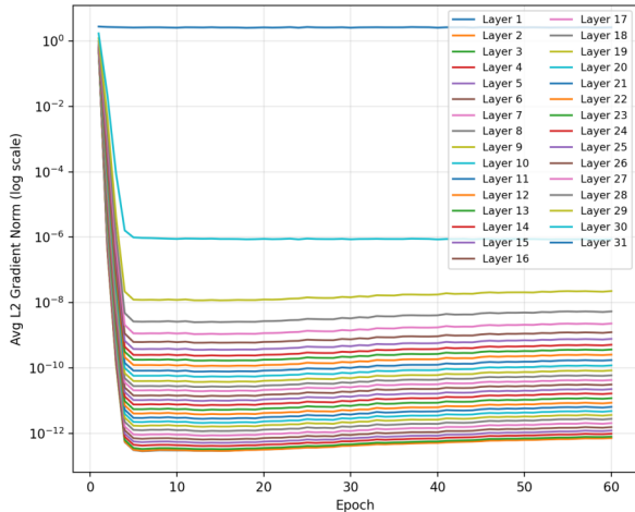
BP Gradient Norms
