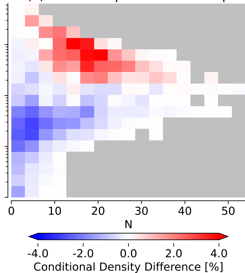
(d) Rain at Ship - No Rain at Ship
