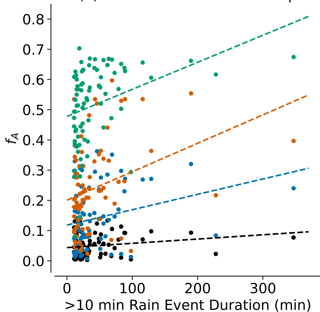
(d) Rain at Ship - No Rain at Ship
