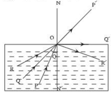
চিত্র ১১.৭ : পূর্ণ অভ্যন্তরীণ প্রতিফলন ও সংকট কোণ
