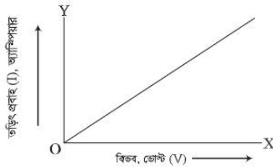
চিত্র ৯.৪ : ও'মের সূত্রের লেখচিত্র
