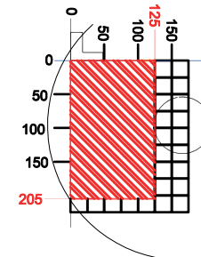
90° : 205 x 125 mm
