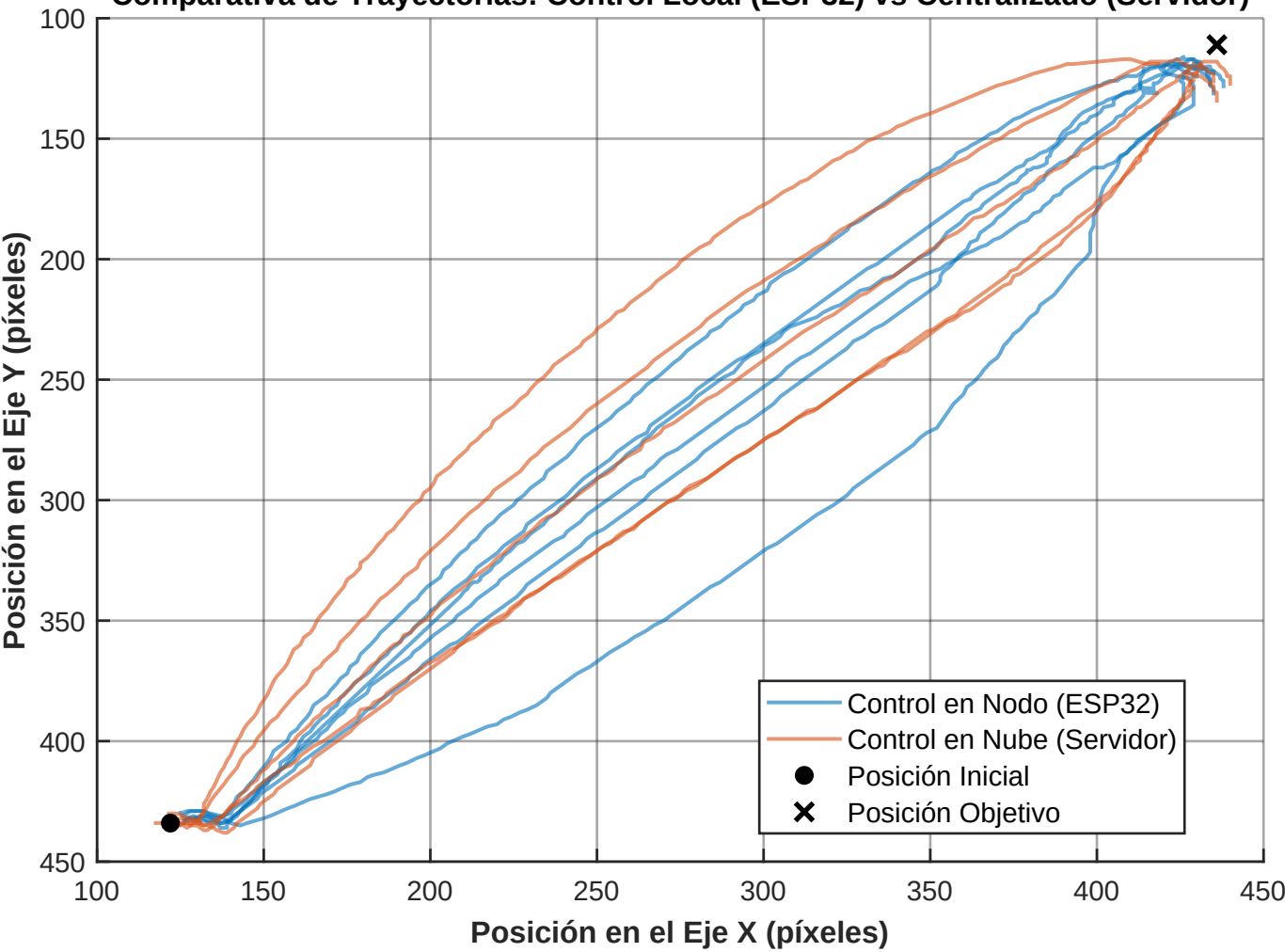
Comparativa de Trayectorias: Control Local (ESP32) vs Centralizado (Servidor)
