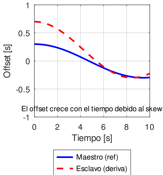
(b) Impacto de la deriva de los relojes
