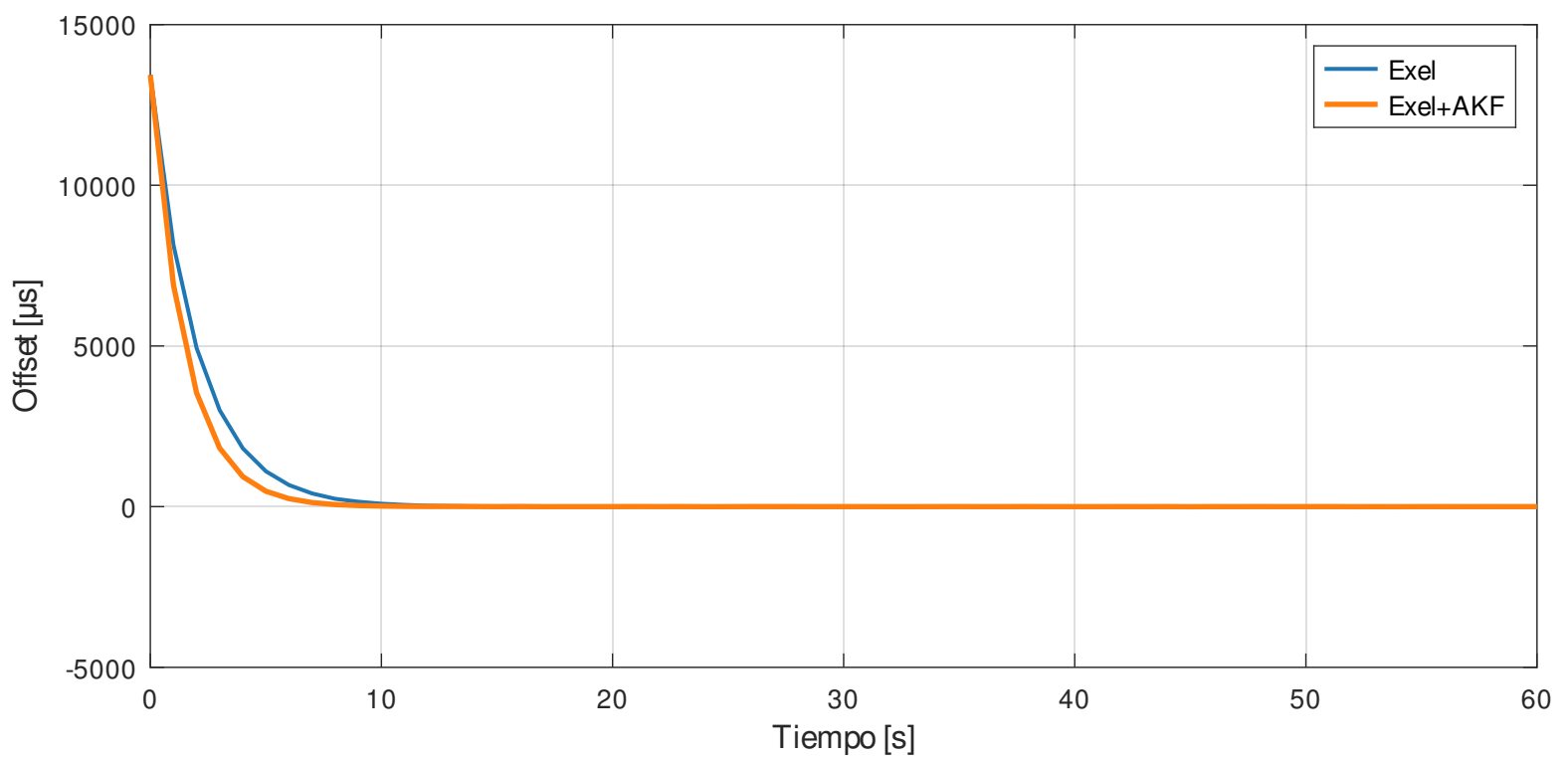
Variación del offset del protocolo gPTP
