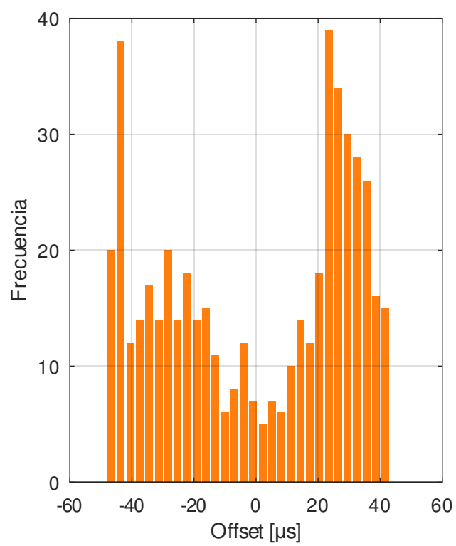
Exel+AKF (mejorado)
