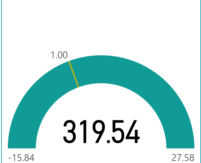
Daily_Return
