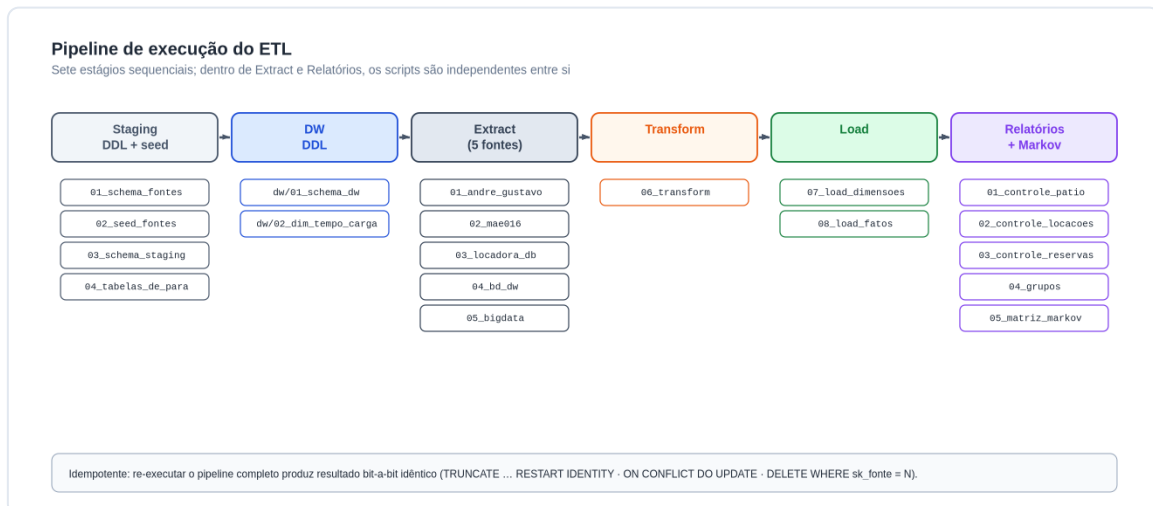
Figura 2. Pipeline resumido do ETL com etapas sequenciais.
