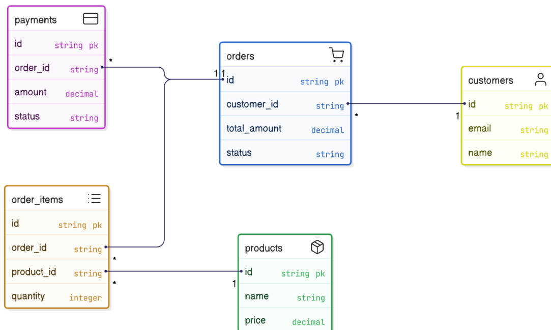
Fig: ERD Diagram
