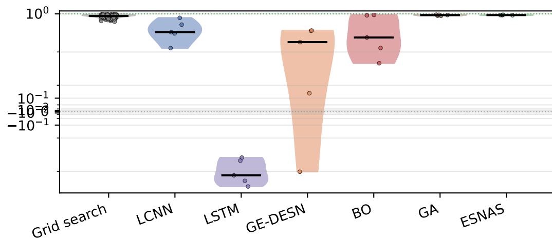
lorenz
