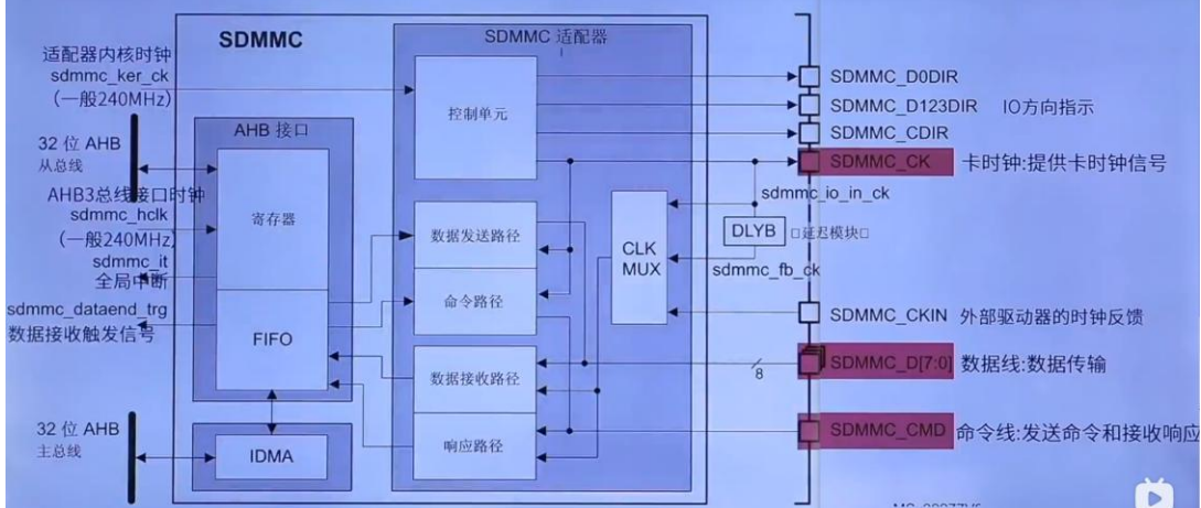
H750 SDMMC框图
