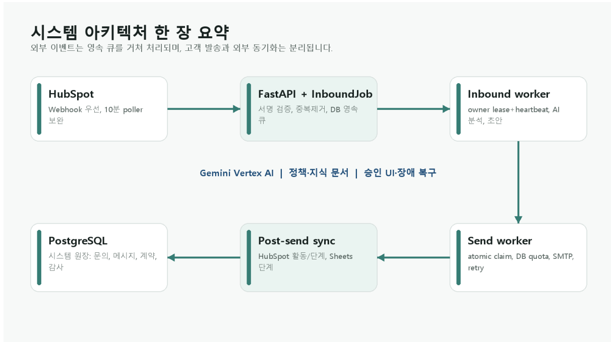
그림 1. Webhook 수신부터 발송 후 동기화까지의 시스템 경계
