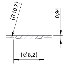
DETAIL Y SCALE 2:1
