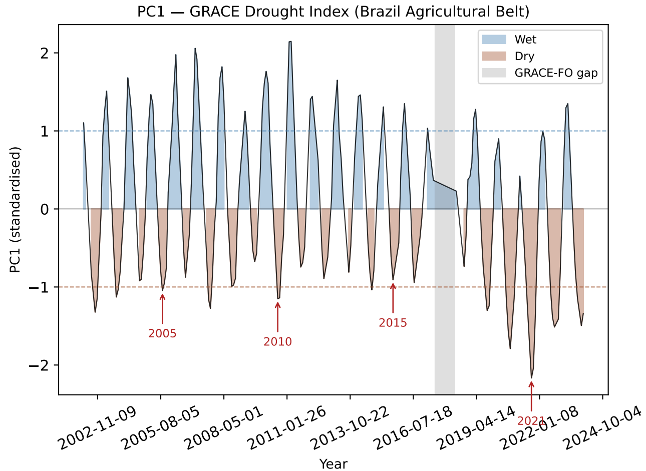
Fig. 2 — GRACE EOF/PCA (2002-2023)
