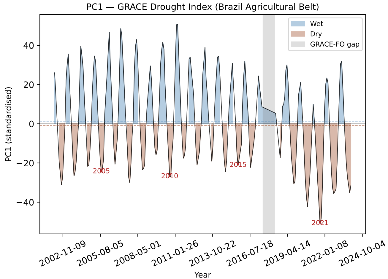
Fig. 2 — GRACE EOF/PCA (2002-2023)
