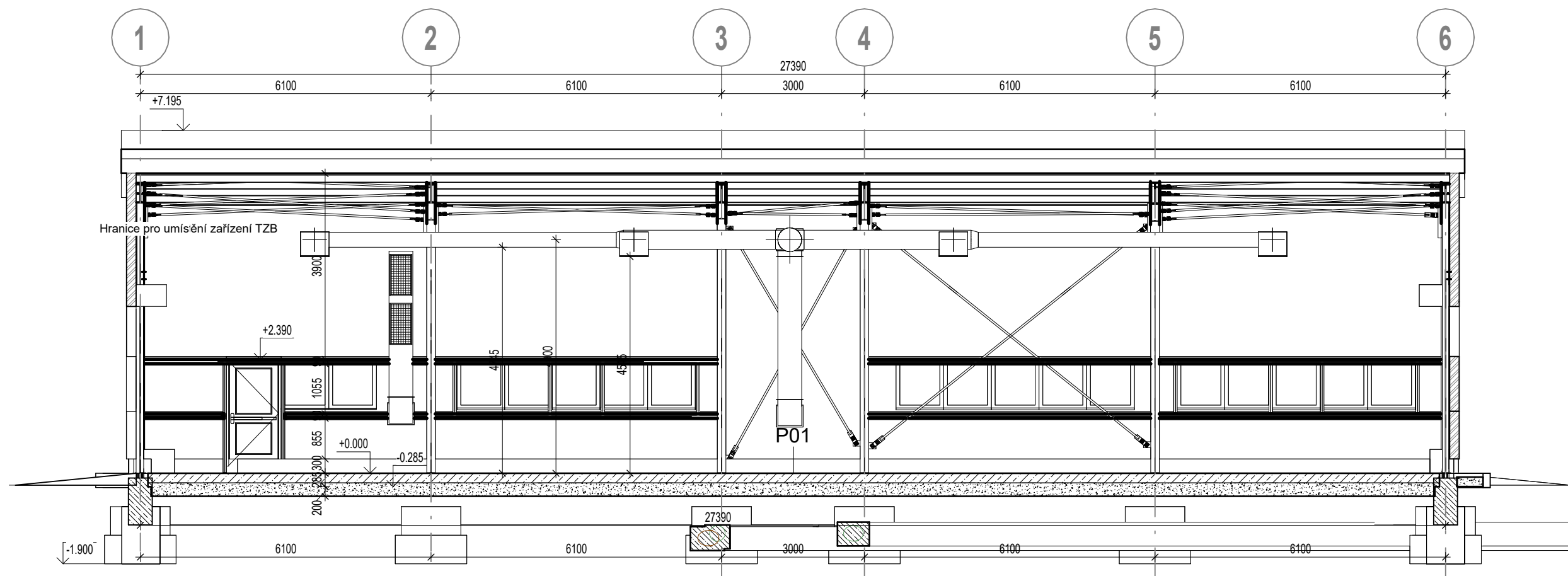
ŘEZ "B"
