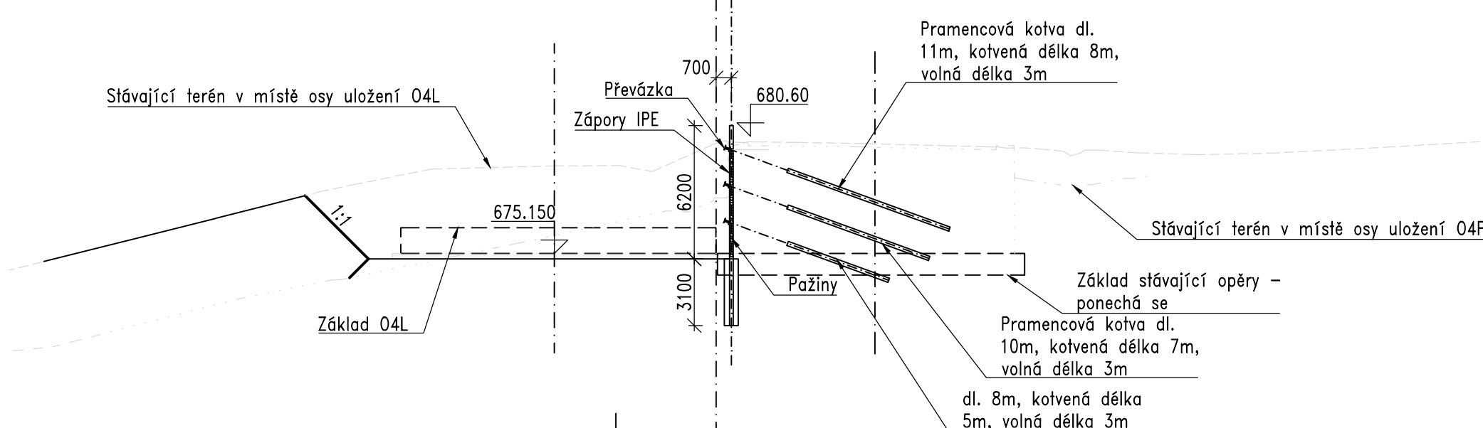
PŘÍČNÝ ŘEZ V OSE ULOŽENÍ 04L 1:100
