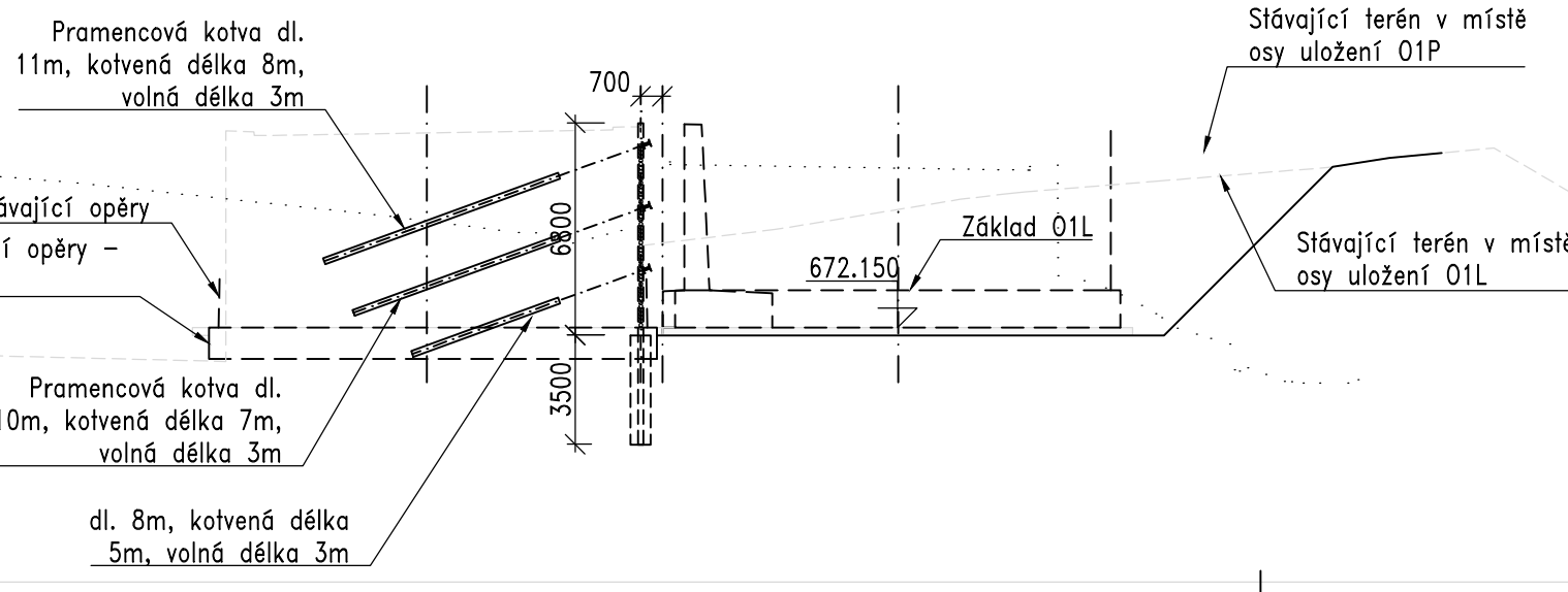
PŘÍČNÝ ŘEZ V OSE ULOŽENÍ 01L 1:250
