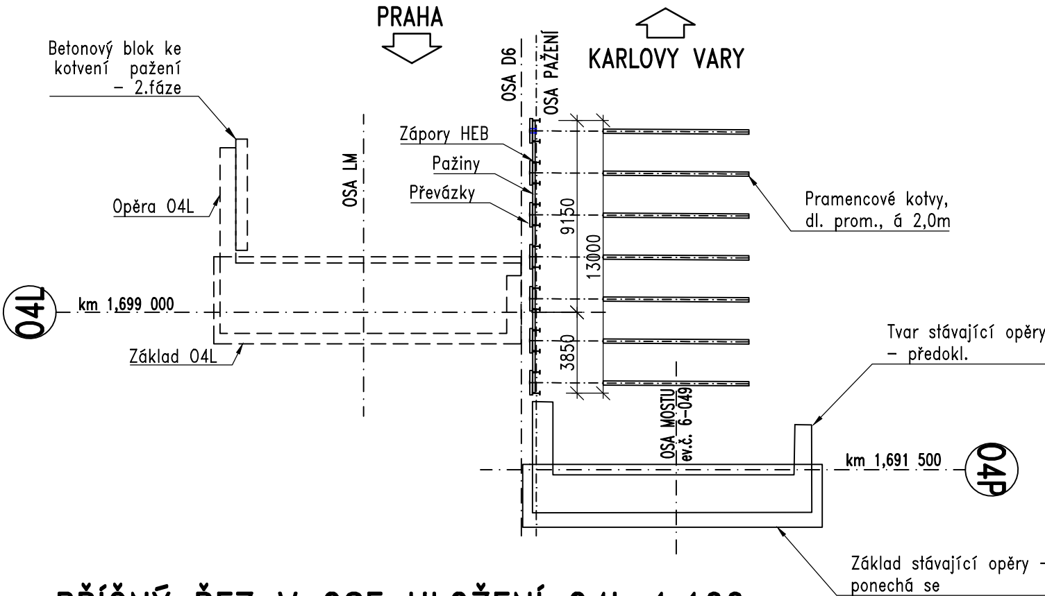
PŘÍČNÝ ŘEZ V OSE ULOŽENÍ 04L 1:100
