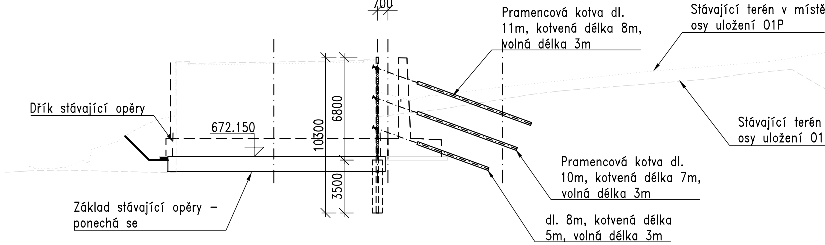
ŘEZ V OSE ULOŽENÍ O1P 1:250
