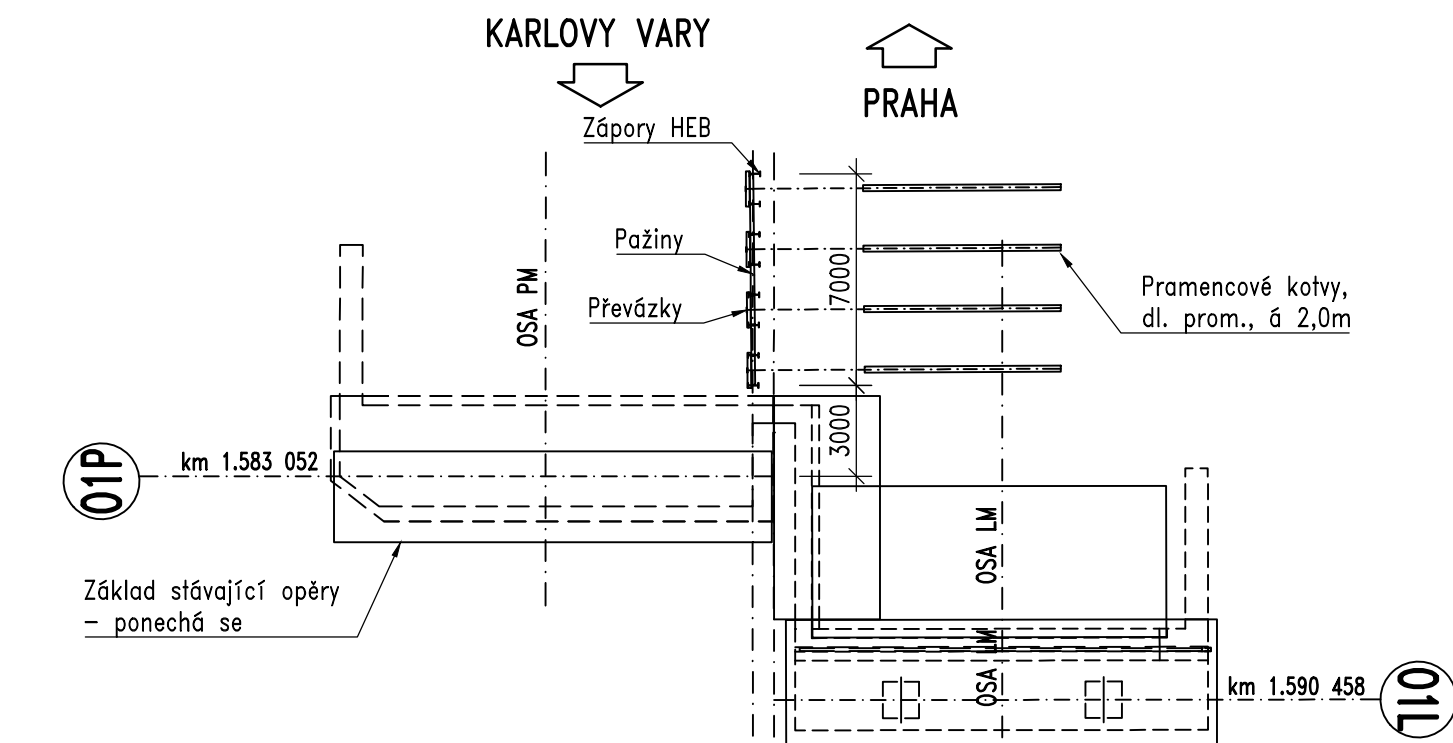
ŘEZ V OSE ULOŽENÍ O1P 1:250
