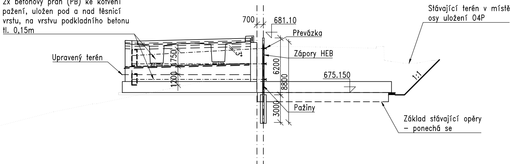
ŘEZ V OSE ULOŽENÍ O4P 1:250
