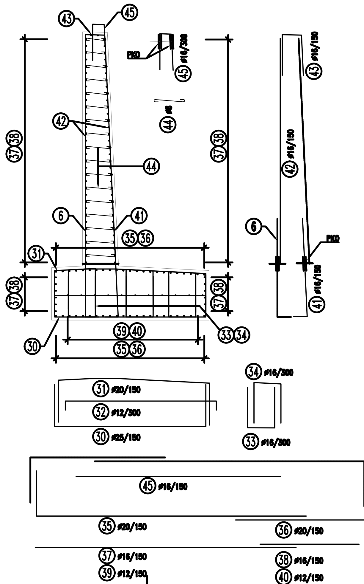
ŘEZ KŘÍDLEM PM 1:50
