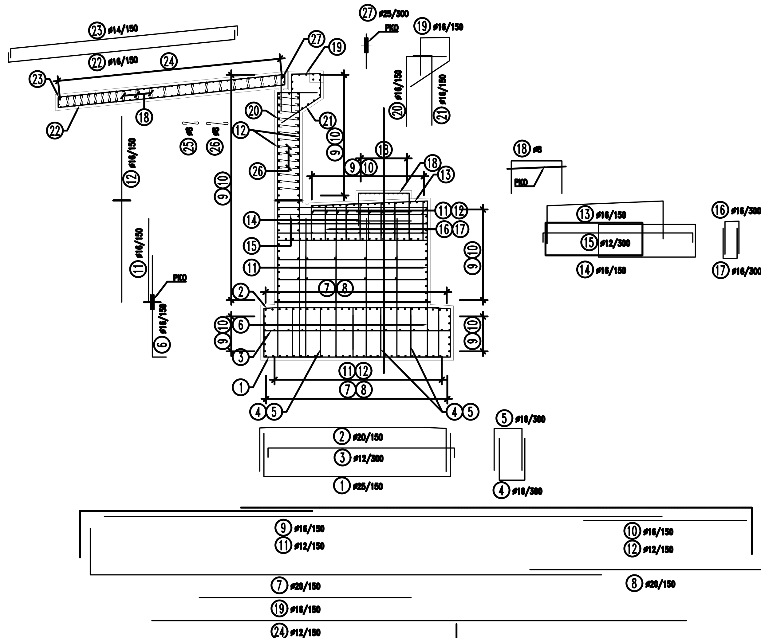
PODÉLNÝ ŘEZ OPĚROU O1 1:50
