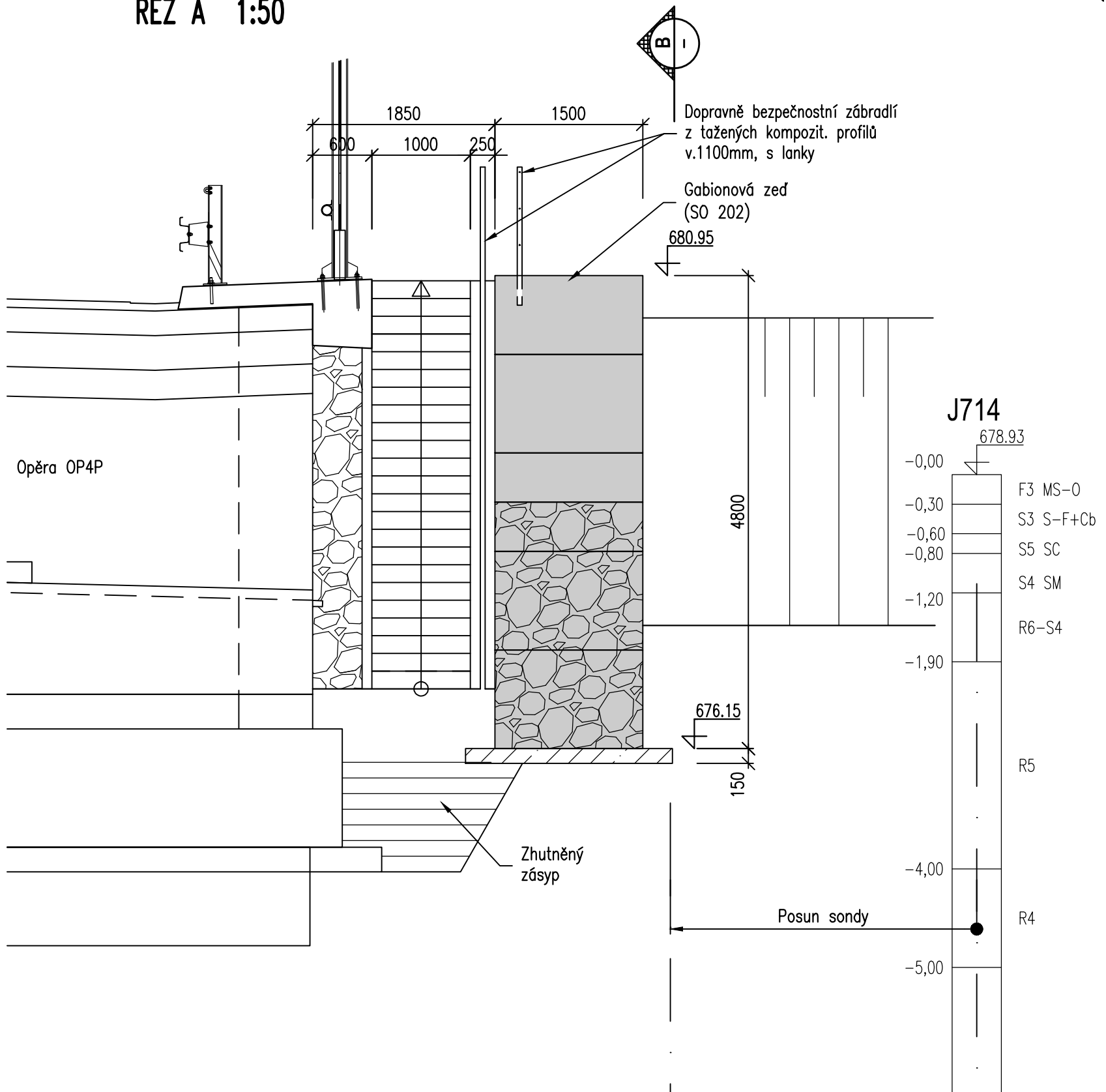
ŘEZ A 1:50
