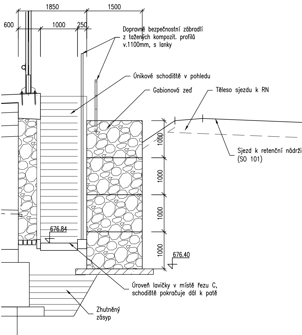
ŘEZ C 1:50
