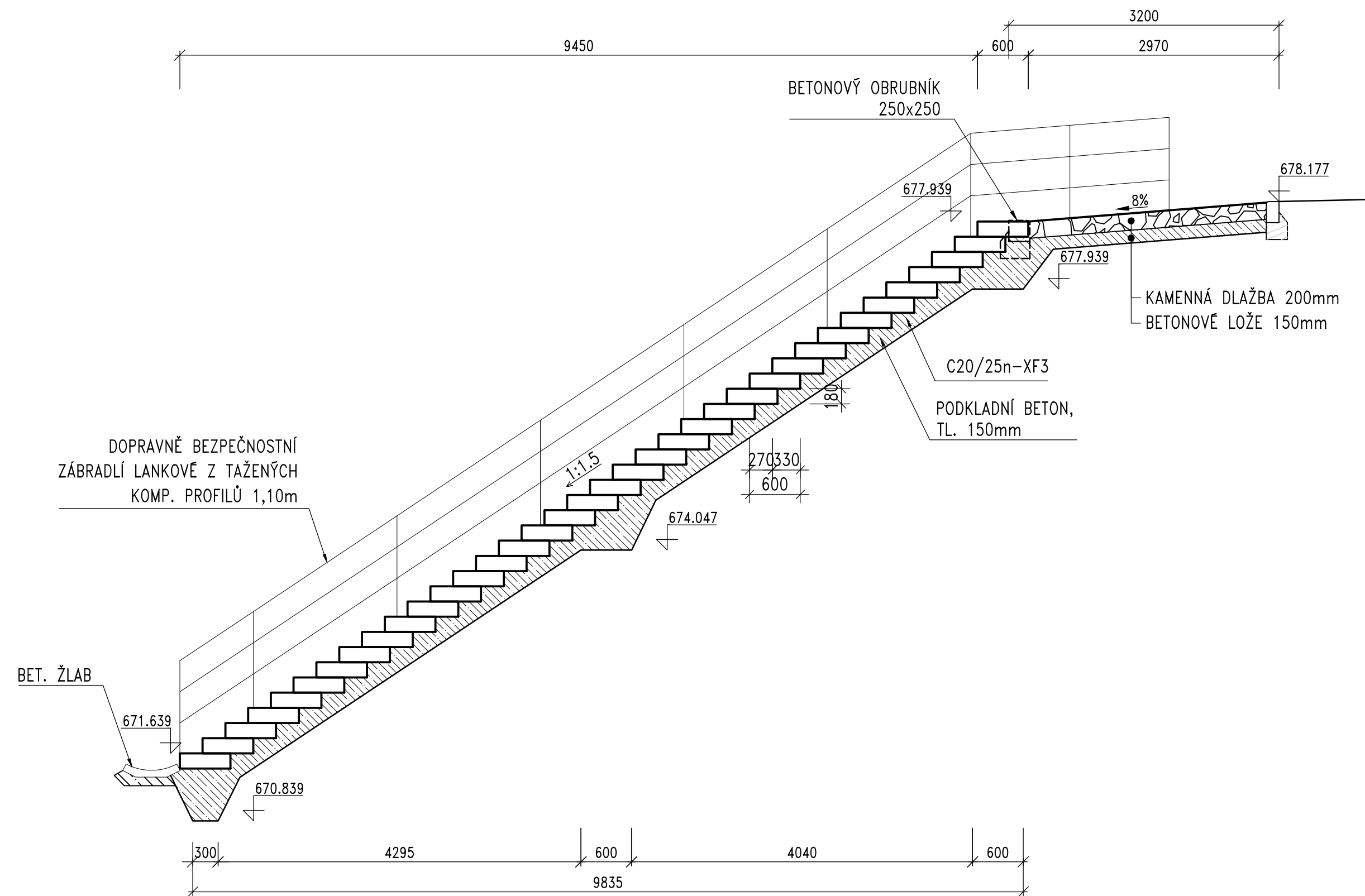
ŘEZ ÚNIKOVÝM SCHODIŠTĚM U 01P 1:50
