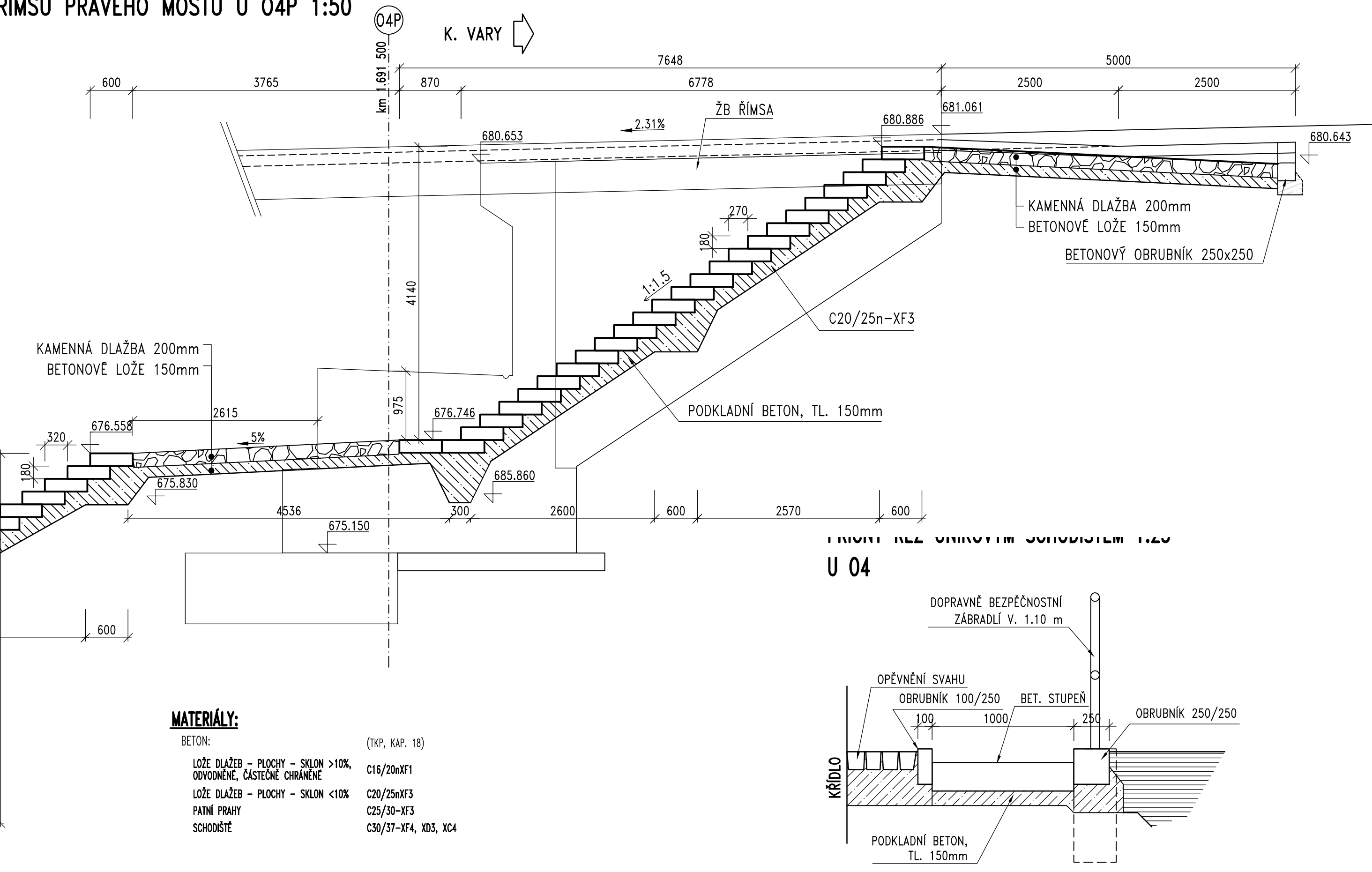
POHLED NA VNĚJŠÍ ŘÍMSU PRAVÉHO MOSTU U 04P 1:50
