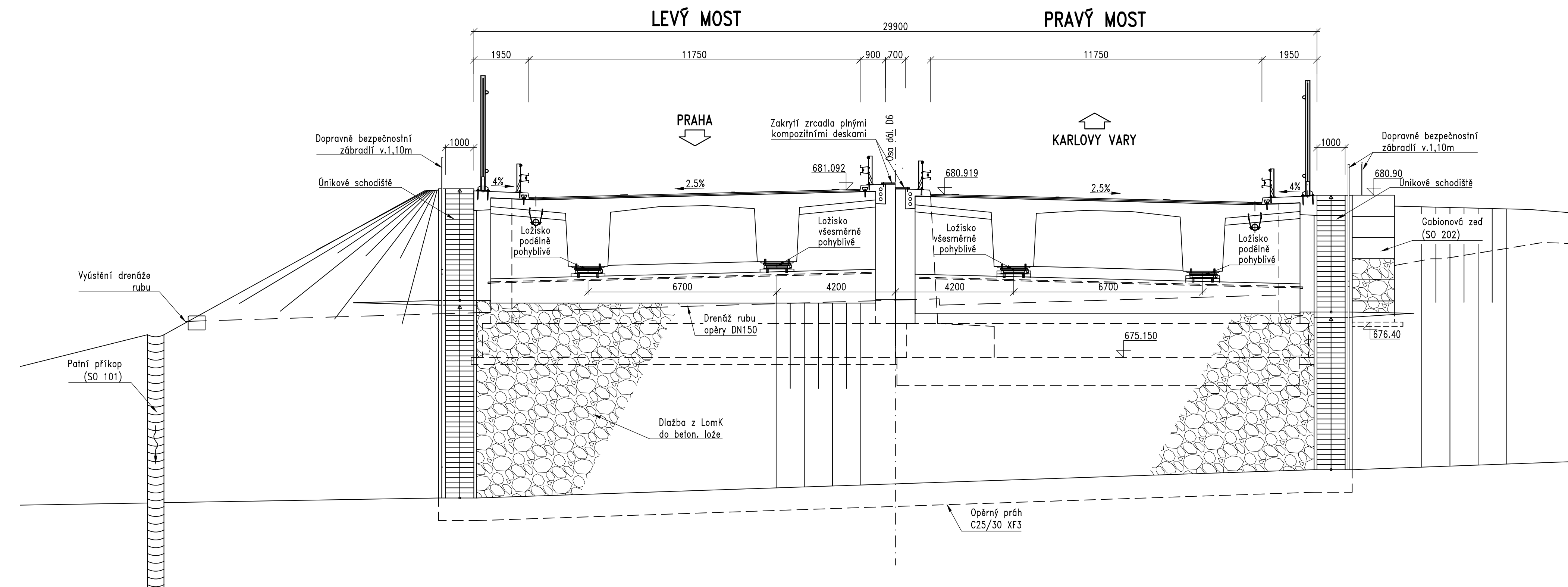
OPĚRA 04L, 04P 1:100
