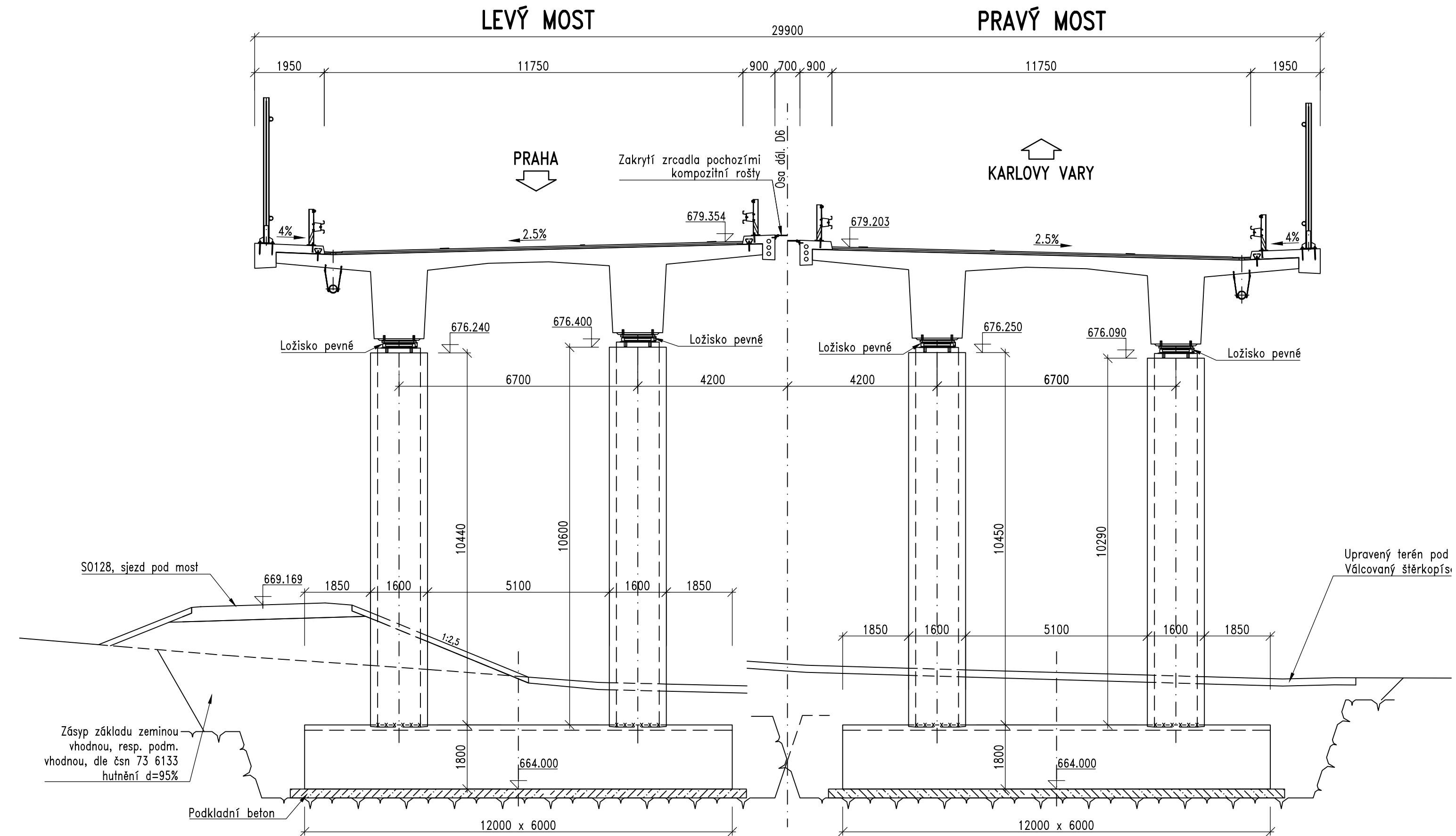
PILÍŘE P2L, P2P 1:100
