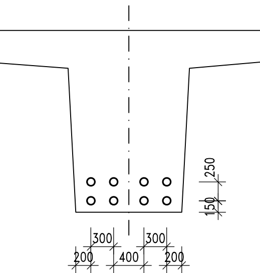
ŘEZ V POLI 1:50
