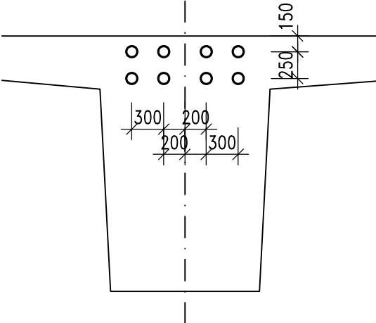
ŘEZ NAD PILÍŘEM 1:50
