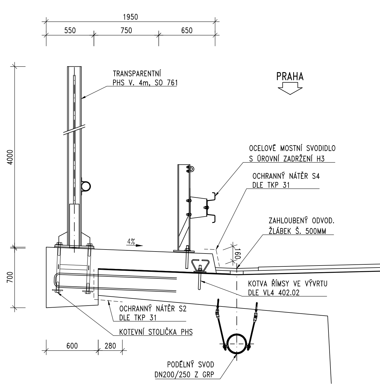
ŘEZ VNĚJŠÍ ŘÍMSOU, PRAVÝ MOST 1:25
