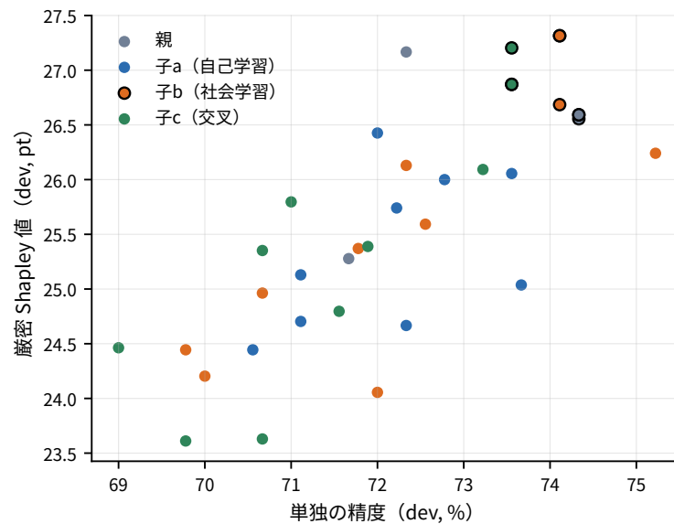
図 5.2: 系統 S の各世代の候補の単独の精度と厳密 Shapley 値 (dev) . 黒い縁は選ばれた候補
