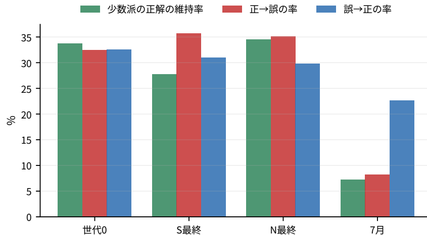
図 5.5: 議論の正誤の遷移. 少数派の正解の維持率は、round0 で 1 体だけが正解していた問題でその正解が保たれた割合. 正→誤と誤→正は、議論した問題でのエージェントごとの遷移の割合
