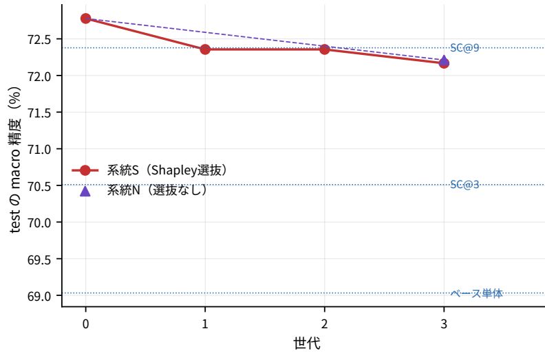
図 5.3: 系統ごとの test の macro 精度の推移. 点線はベースモデルの基準
