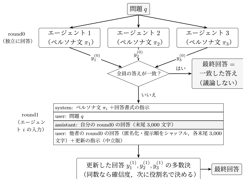
図 3.2: 議論の Protokol. round0 の答えが全員一致した問題では議論を省く (3.3.3 項). round1 では, 自分の round0 の回答を会話履歴に保持したまま他者の回答を読む.
