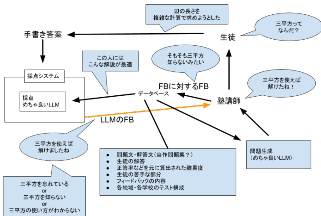
図2 提案システムの全体像：採点→DB蓄積→フィードバック→問題生成のサイクル
