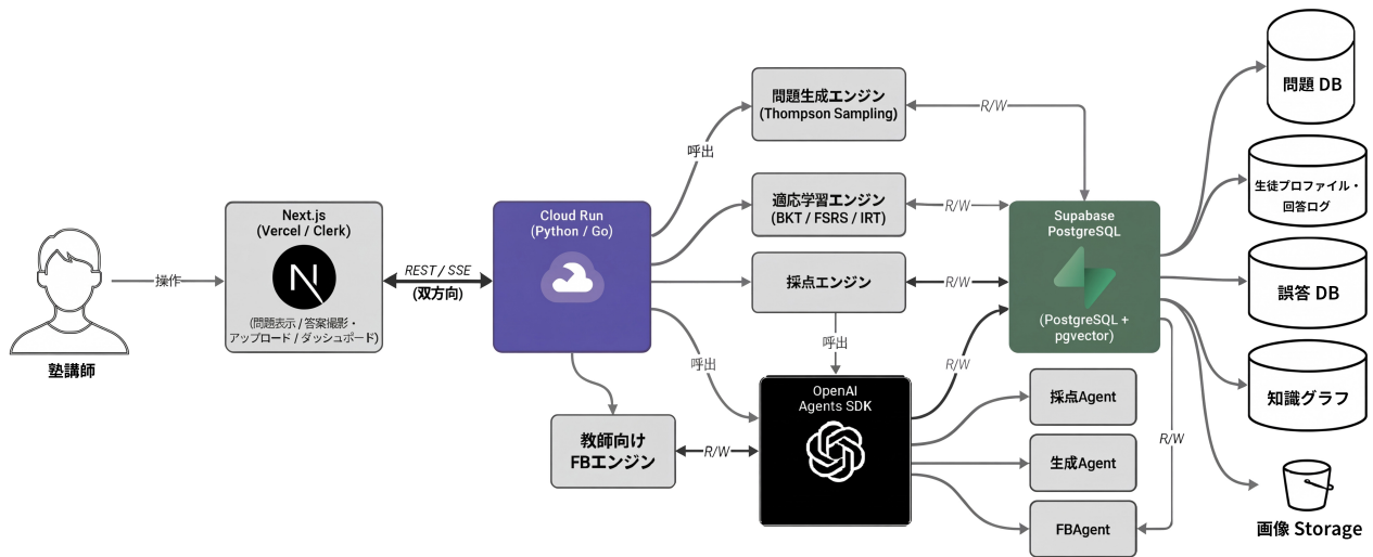
図3 システム構成図：フロントエンド・バックエンド・AI Agent・データベースの全体構成
