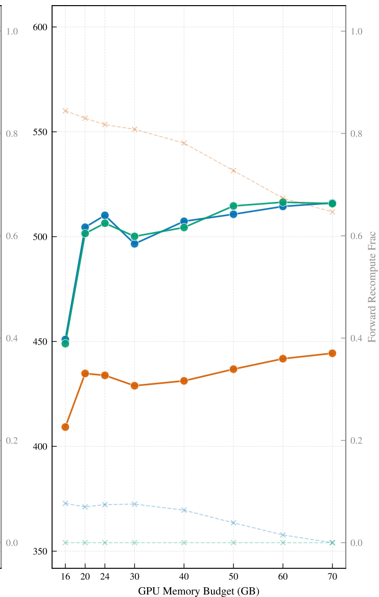
Llama3 8B, SeqLen 64K
