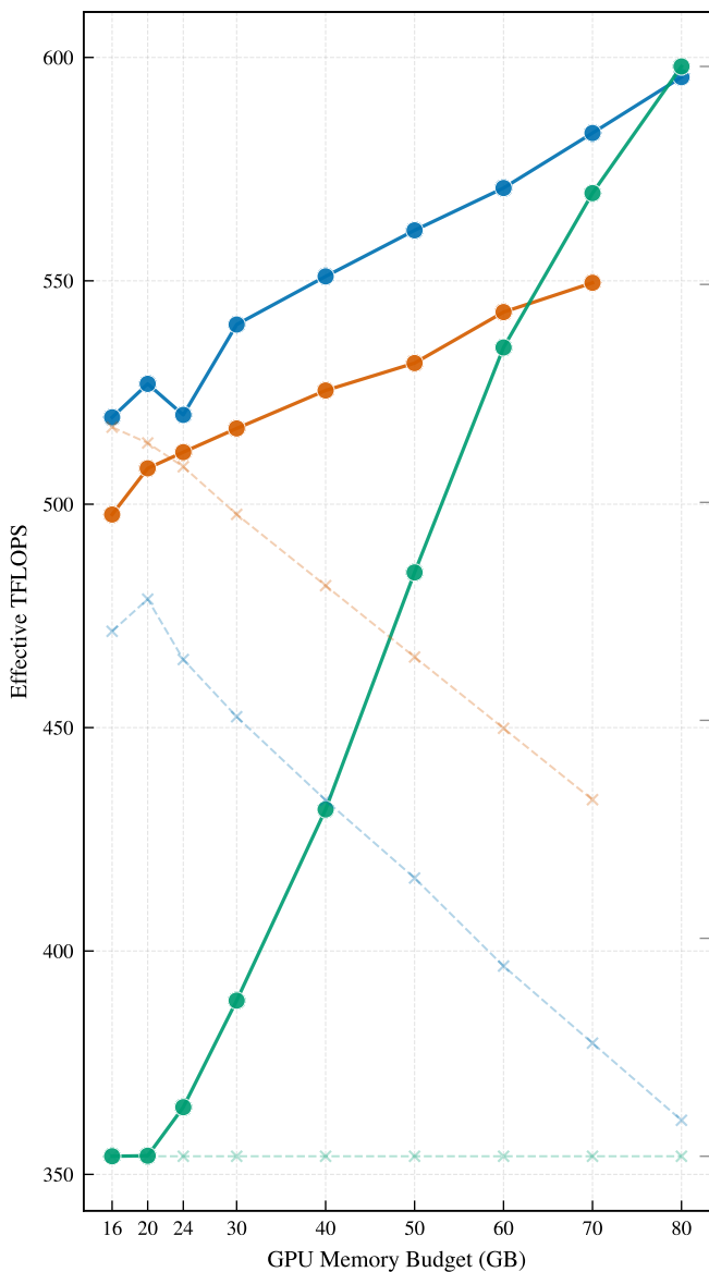
Llama3 8B, SeqLen 1K
