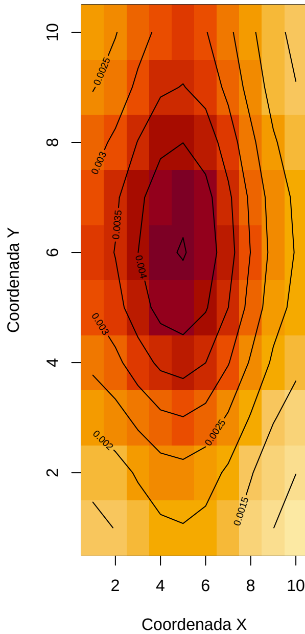
Analítico (Fisher-KPP)
