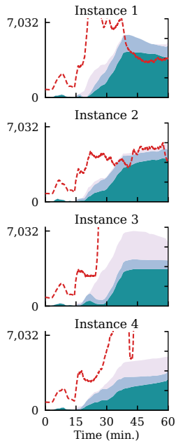
vLLM-router
