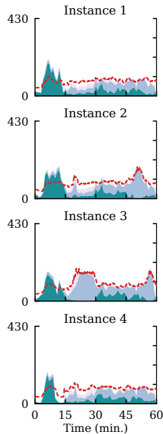
llm-d
