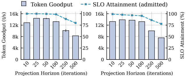
(a) Llama-3.1-70B
