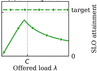
(d) Over-rejection
