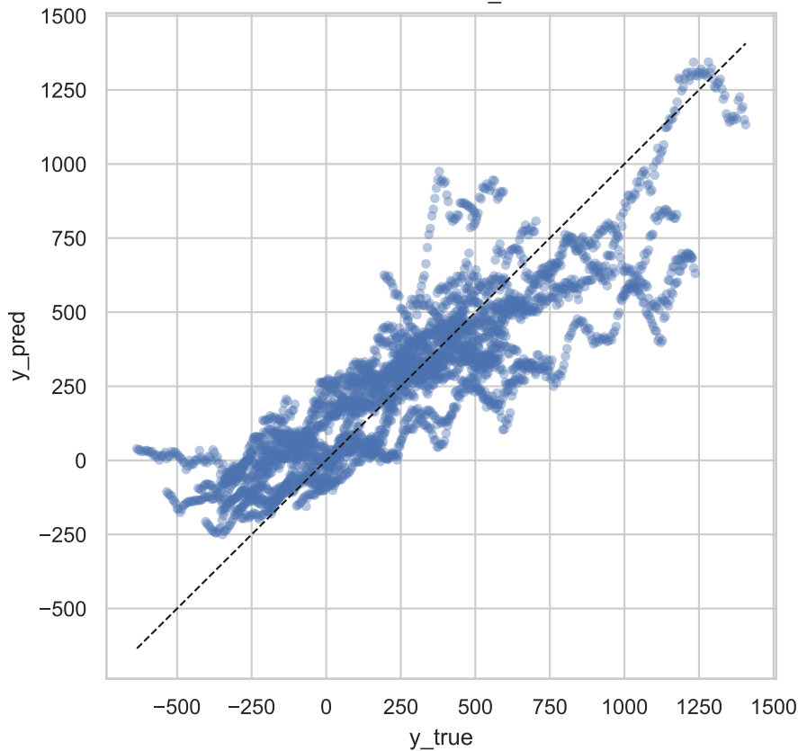
Pred vs GT — Lin15_c71dad01
