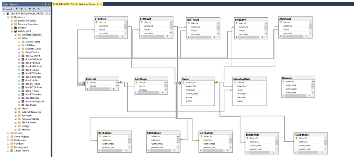
Veritabanı Diyagramı
