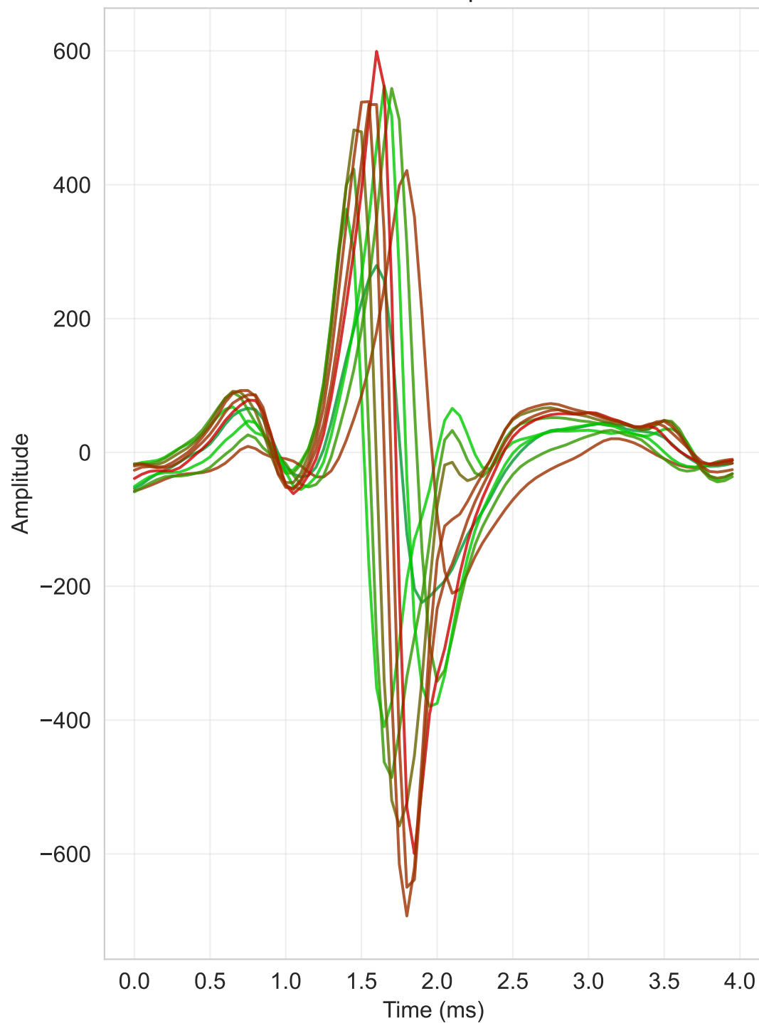
Unit 9 Template
