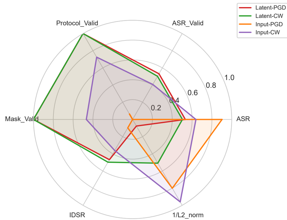
CNN
