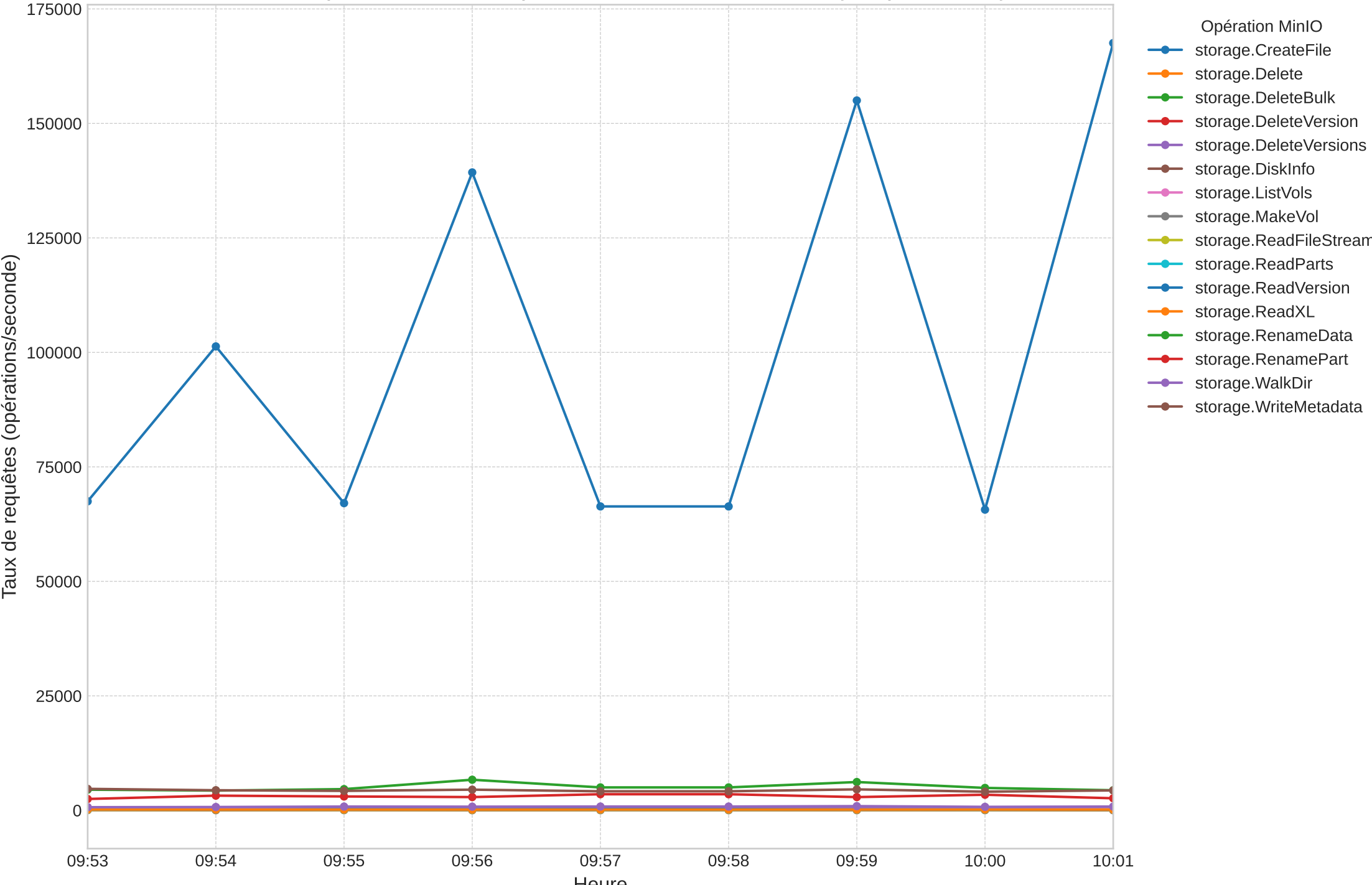
Débit des opérations MinIO pour le backend RocksDB (Requête Q11)
