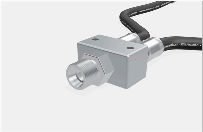
Detalhe ① — Entrada DKO TB22 macho Rosca externa M30×2 (série L) com cone interno 24°.
