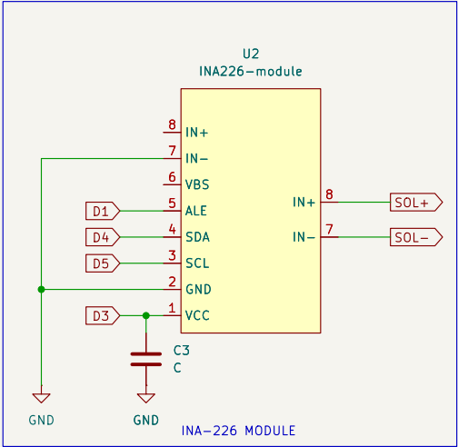
INA-226 MODULE
